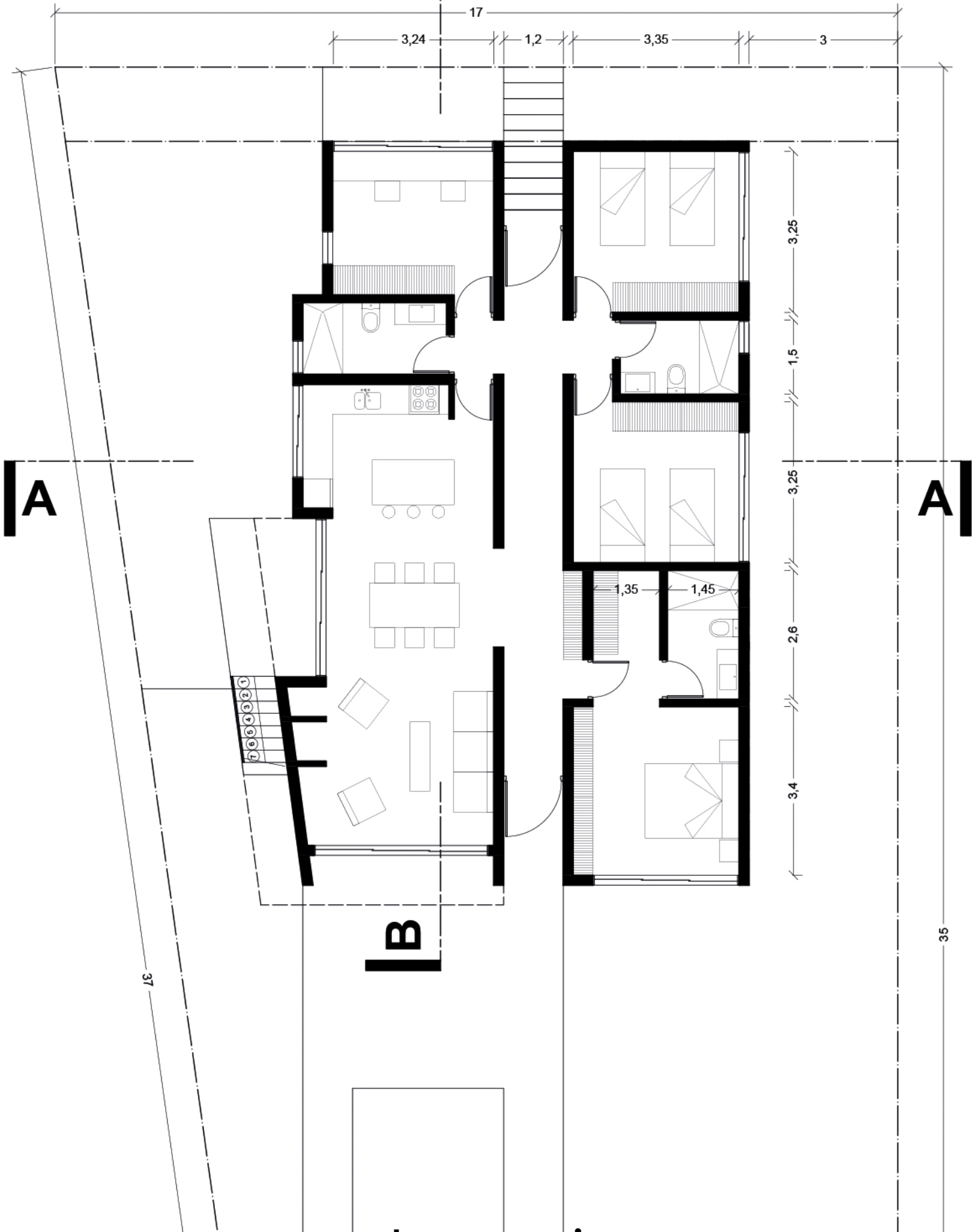
Planta Baja
